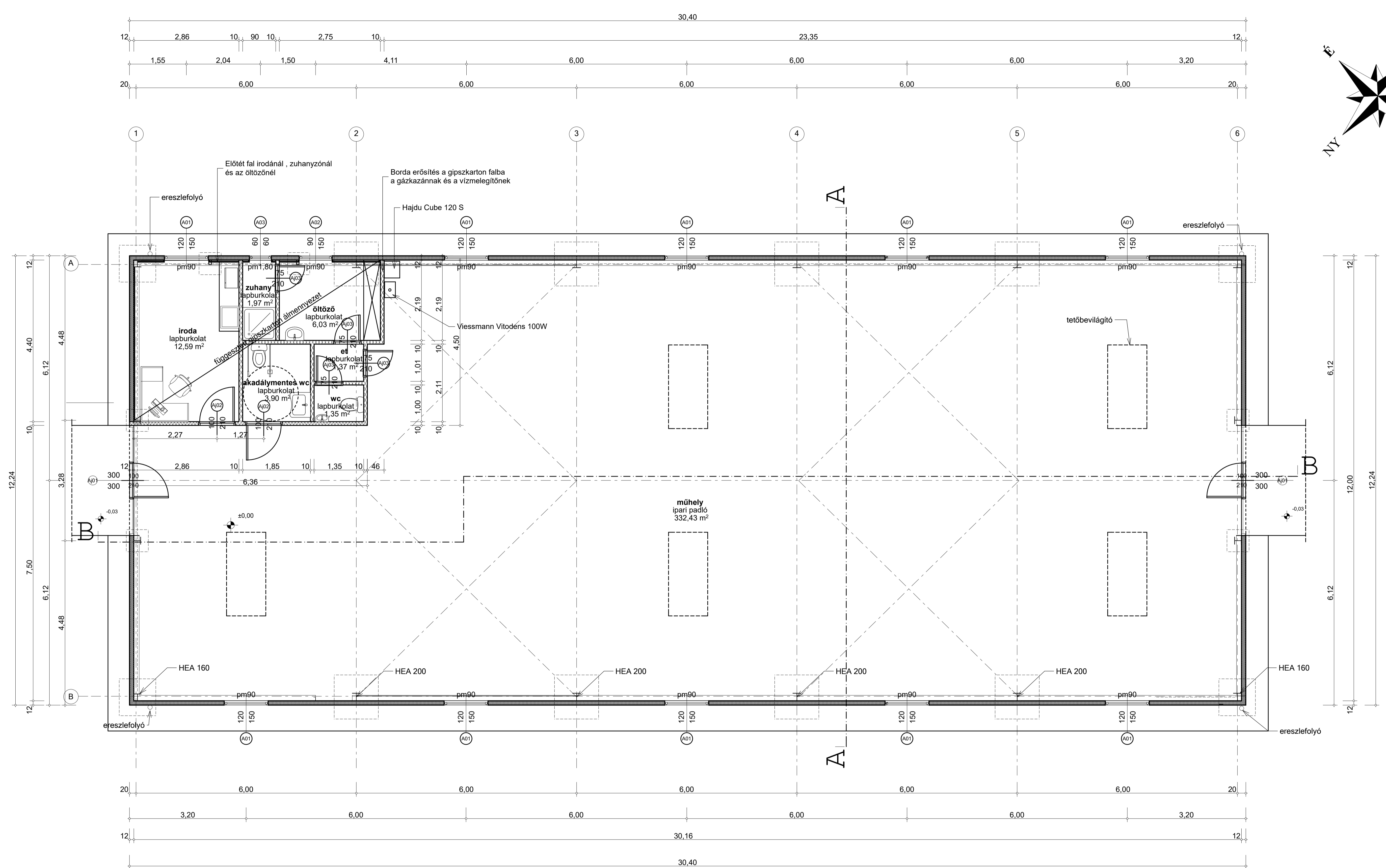
ALAPRAJZ M=1:50
